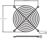
6G-4E for 120mm fan
