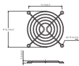
6G-3E for 80mm fan
